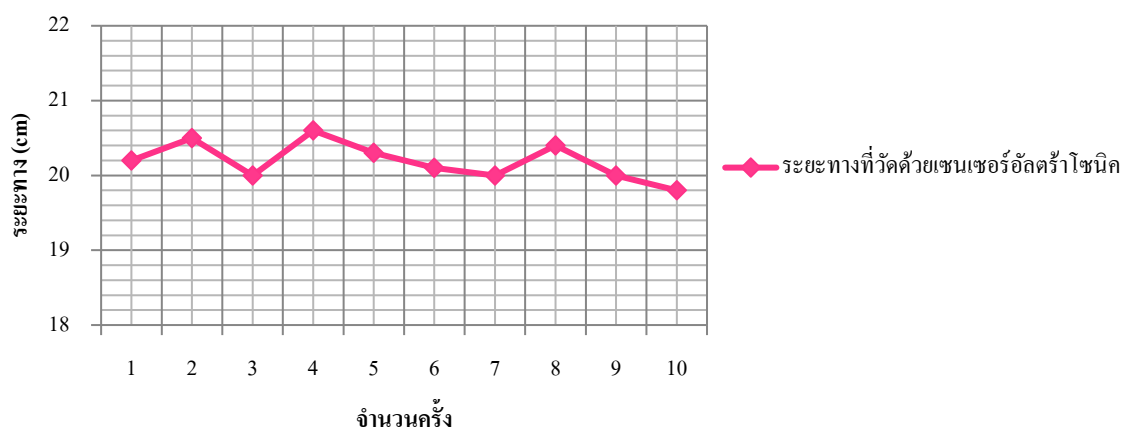
ภาพที่ 6 เปรียบเทียบระยะทางที่วัดด้วยตลับเมตรและจากเซนเซอร์อัลตราโซนิกที่ระยะ 20 เซนติเมตร
