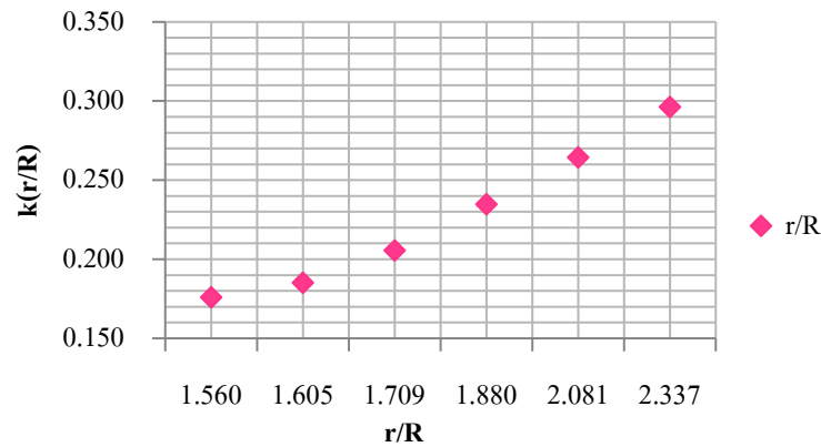
ภาพที่ 12 อัตราส่วนระหว่าง \left(\frac{r}{R}\right) กับค่าอิทธิพลของผนังท่อ k\left(\frac{r}{R}\right)
