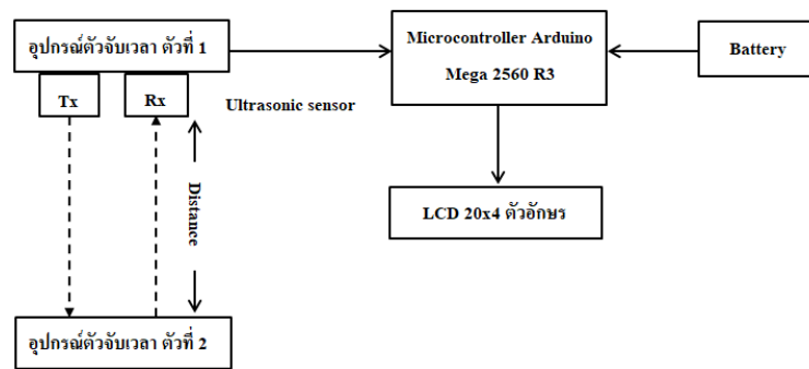
ภาพที่ 4 หลักการทำงานในการวัดระยะทางการเคลื่อนที่ของลูกกลมโลหะ
