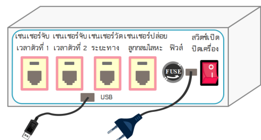
(ค) ด้านหลังของกล่องควบคุมการทำงาน
