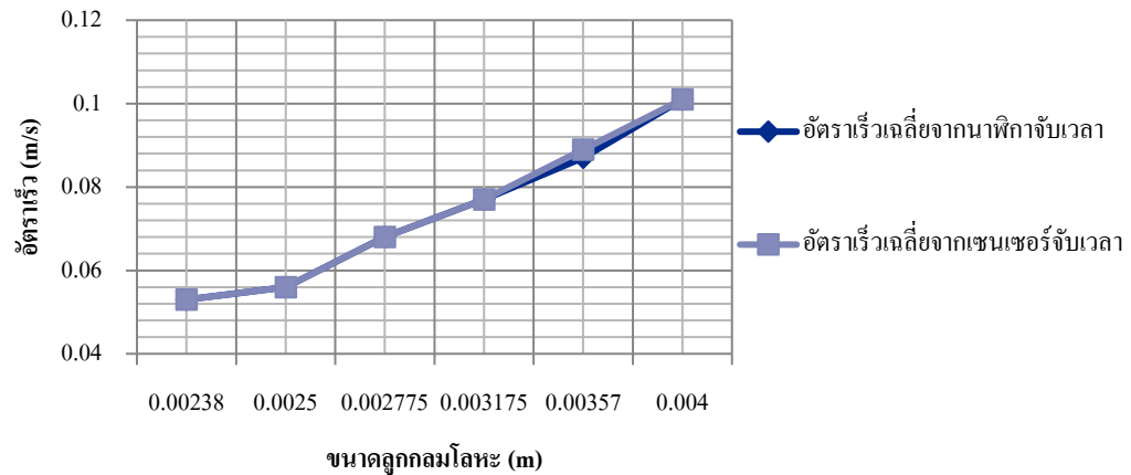
ภาพที่ 11 อัตราเร็วเฉลี่ยจากนาฬิกาจับเวลา และจากเซนเซอร์จับเวลาจากการเคลื่อนที่ของลูกกลมโลหะแต่ละลูก ที่ระยะ 20 เซนติเมตร
