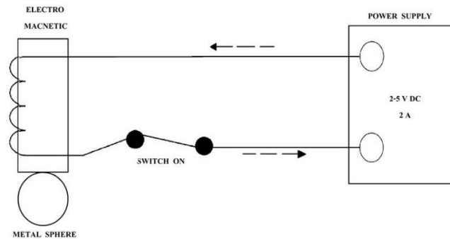
ภาพที่ 1 หลักการทำงานของชุดปล่อยลูกกลมโลหะ
