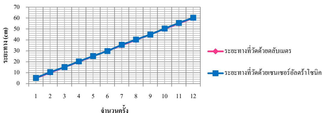
ภาพที่ 7 ความสัมพันธ์ระหว่างระยะทางที่วัดด้วยตลับเมตรและเซนเซอร์อัลตราโซนิก
