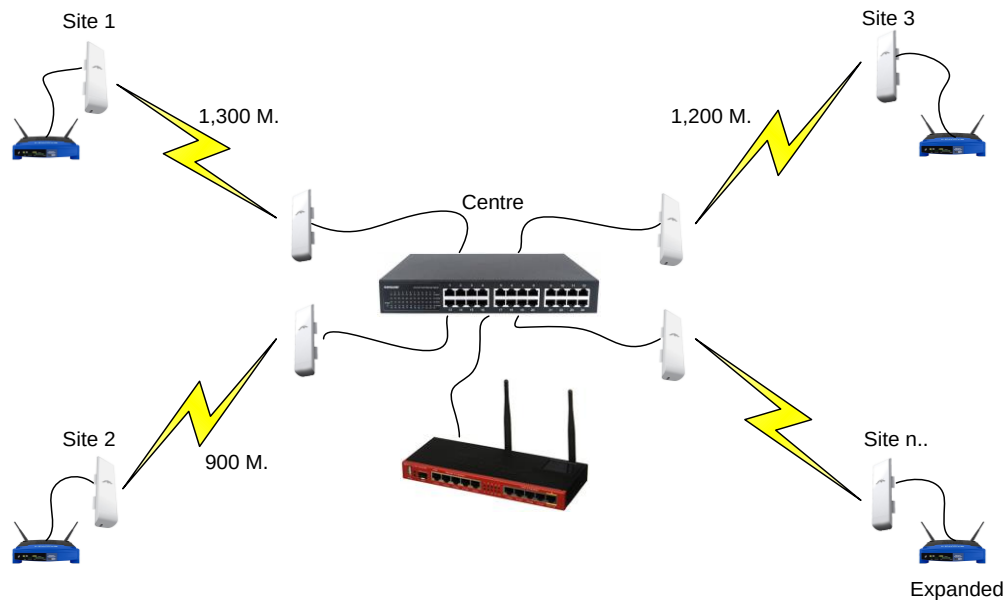
ภาพที่ 2 แสดงแผนผังระบบเครือข่ายอินเทอร์เน็ตของชุมชน
