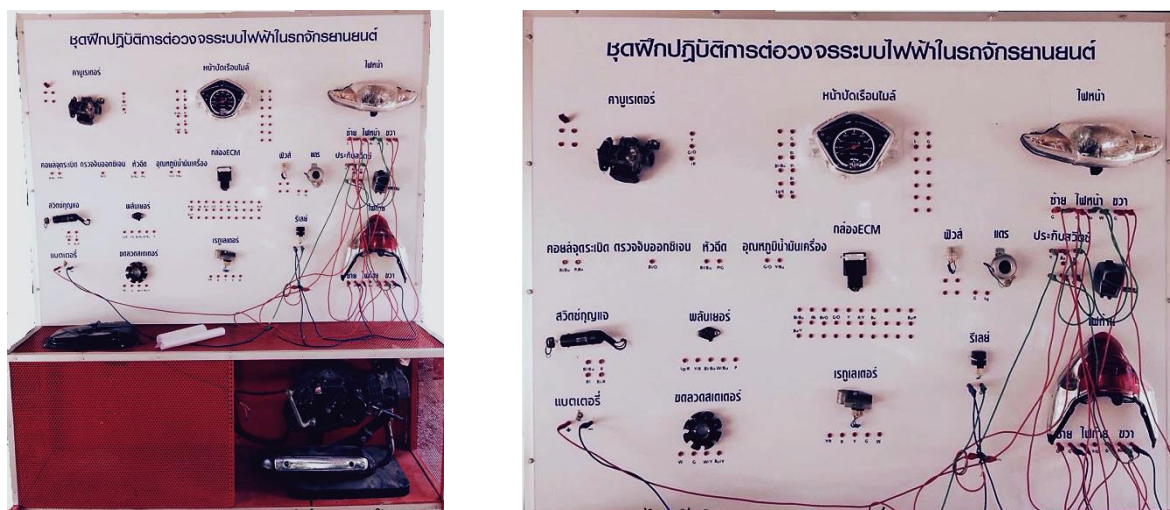
รูปที่ 1 ชุดฝึกปฏิบัติการต่อวงจรระบบไฟฟ้าในรถจักรยานยนต์
