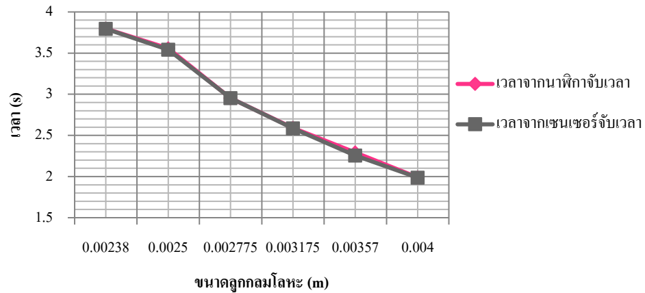
ภาพที่ 10 เวลาจากนาฬิกาจับเวลา และจากเซนเซอร์จับเวลาจากการเคลื่อนที่ของลูกกลมโลหะแต่ละลูก ที่ระยะ 20 เซนติเมตร
